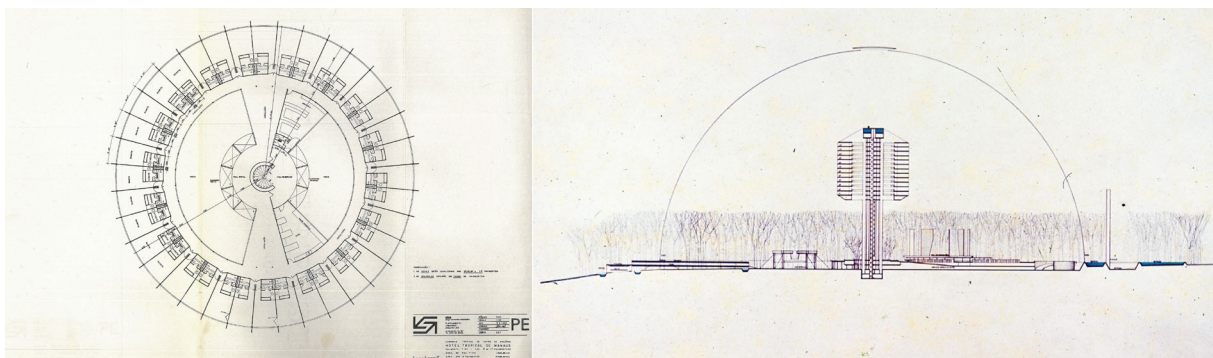
Figura 02 Planta do pavimento tipo e Corte Geral do Tropical Hotel de Manaus Fonte: LEONE, 1969
