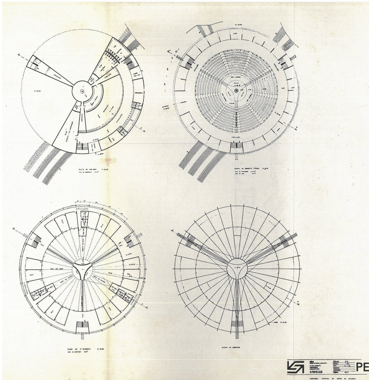
Figura 03 Plantas do Centro de Convenções do Tropical Hotel de Manaus Fonte: LEONE, 1969
