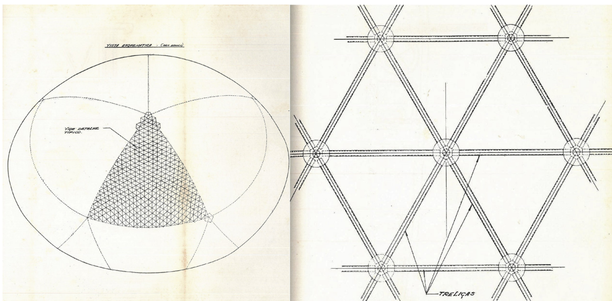
Figura 10 Desenhos Estrutura Domo Tropical Hotel de Manaus Fonte: LEONE, 1969
