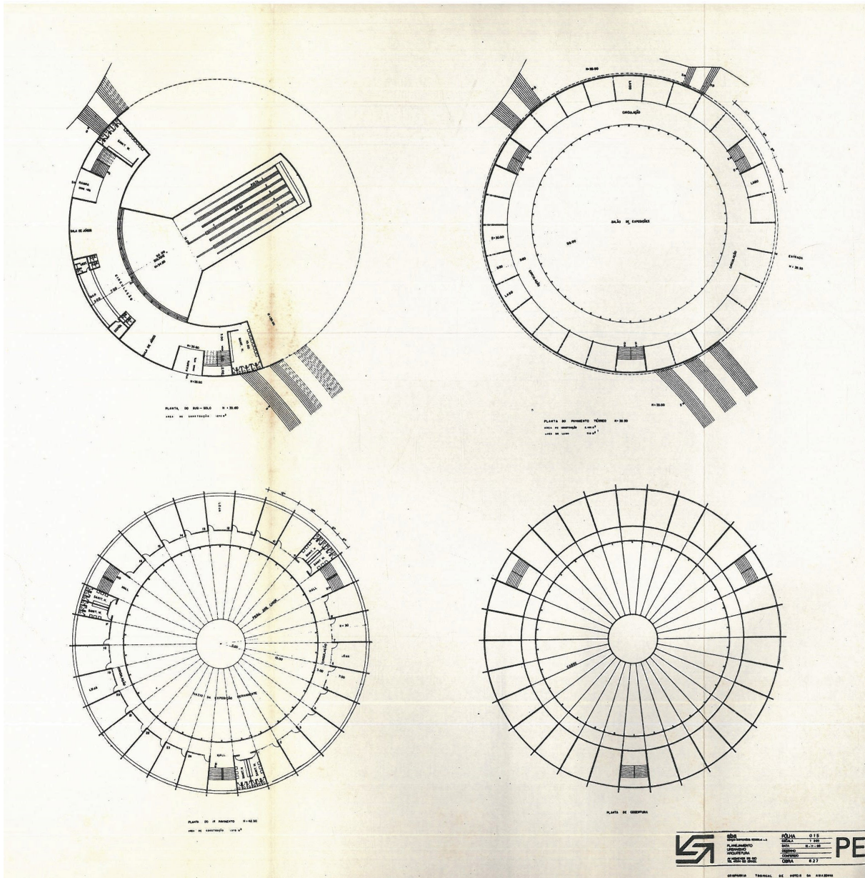
Figura 04 Plantas do Salão de Exposições do Tropical Hotel de Manaus Fonte: LEONE, 1969
