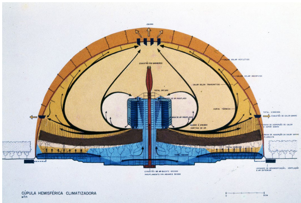
Figura 11 Esquema de Climatização do Tropical Hotel de Manaus Fonte: http://www.bernardesarq.com.br/pt-br/projeto/tropical-de-manaus-domus
