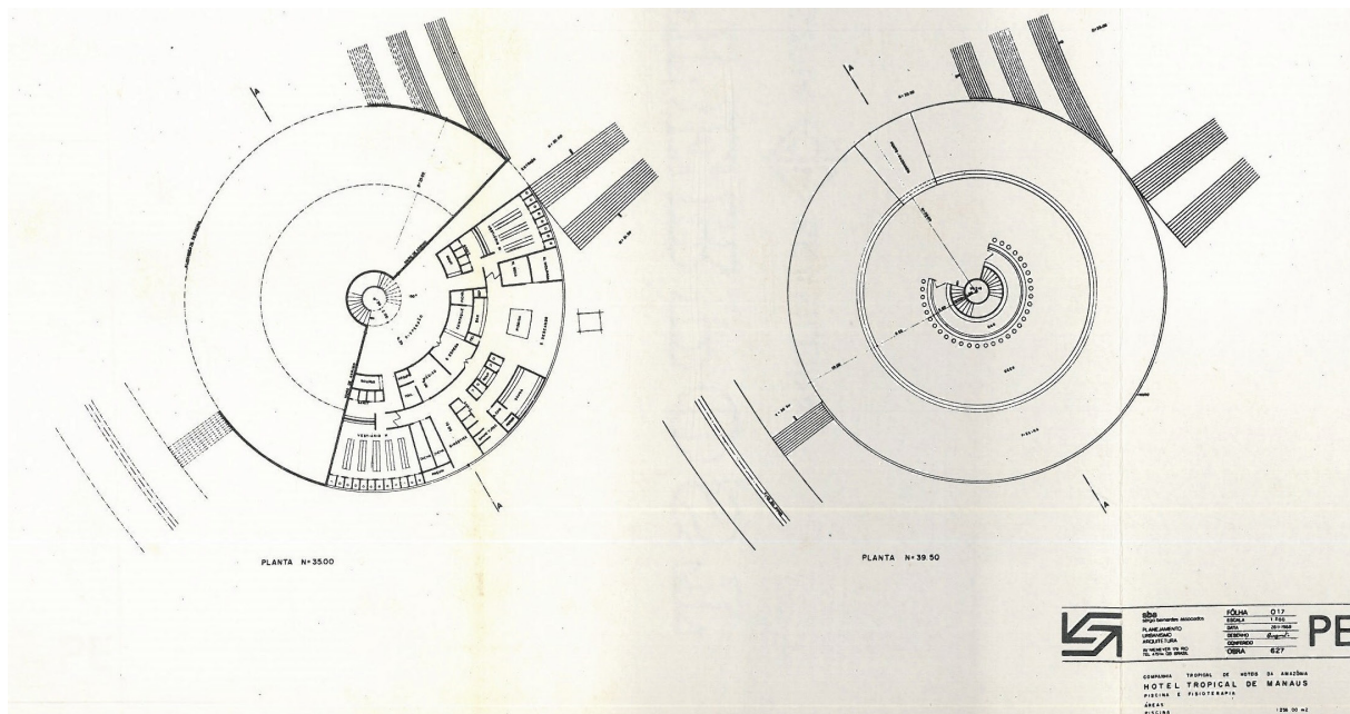
Figura 06 Plantas do Conjunto Bar-piscina-fisioterapia do Tropical Hotel de Manaus Fonte: LEONE, 1969
