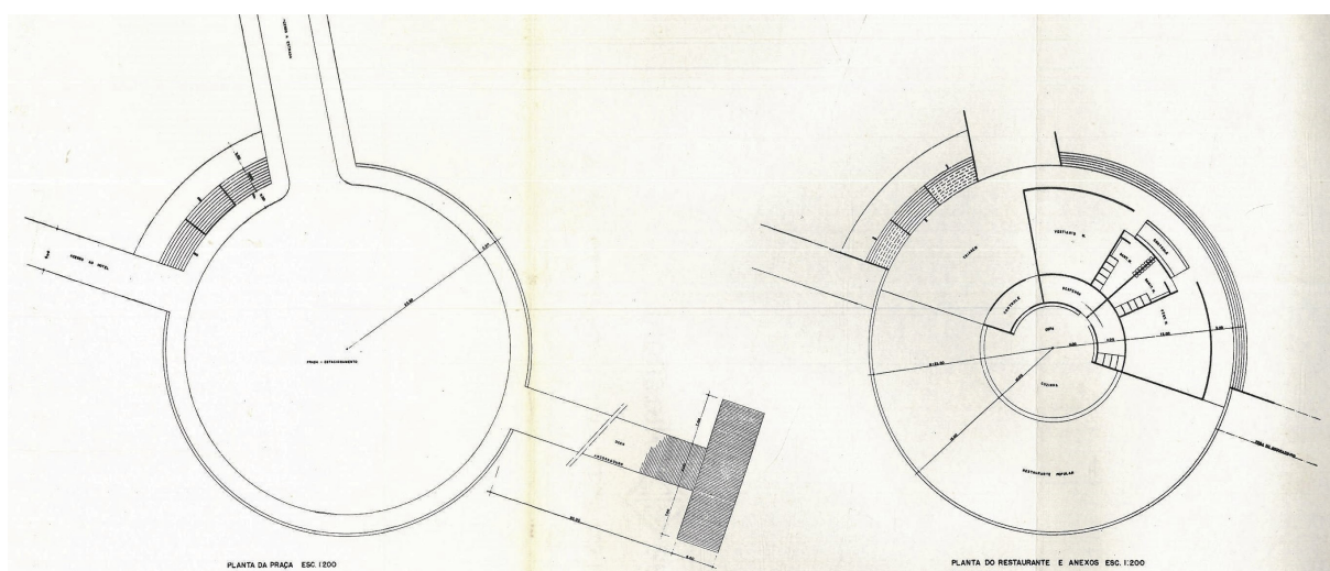
Figura 08 Plantas do Conjunto Boate-piscina-aquário do Tropical Hotel de Manaus Fonte: LEONE, 1969
