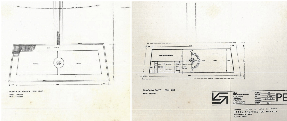
Figura 07 Plantas do Conjunto Boate-piscina-aquário do Tropical Hotel de Manaus Fonte: LEONE, 1969
